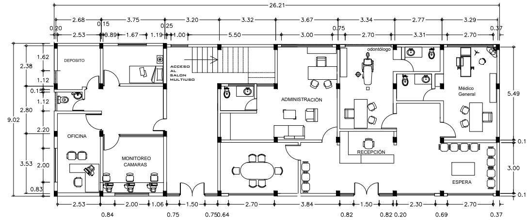
PLANTA BAJA MONITOREO, ADMINISTRACION Y D. MEDICO
