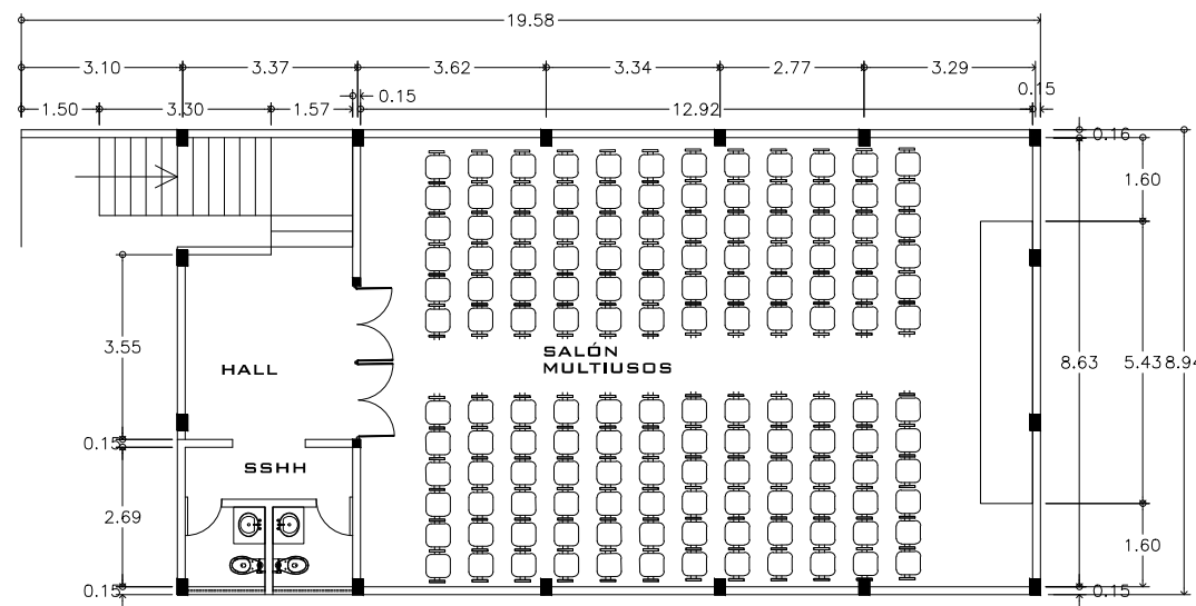
PLANTA ALTA SALÓN MULTIUSO
