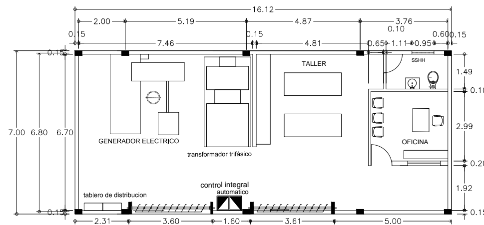
PLANTA BAJA CUARTO DE MAQUINAS
