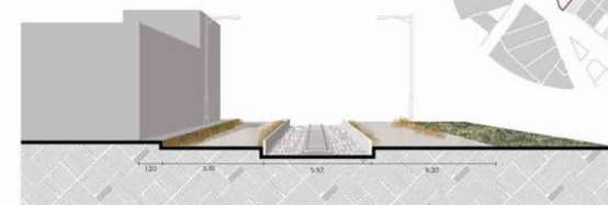
Sección C-C'
