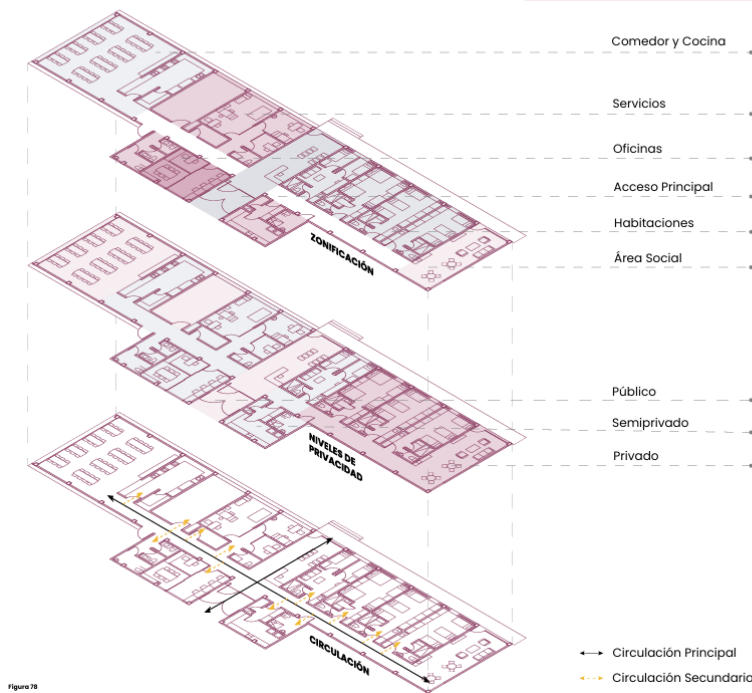
Figura 78 Esquema de organización espacial Casa de Acogida y Comedor Comunitario
