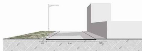
Sección B-B'
