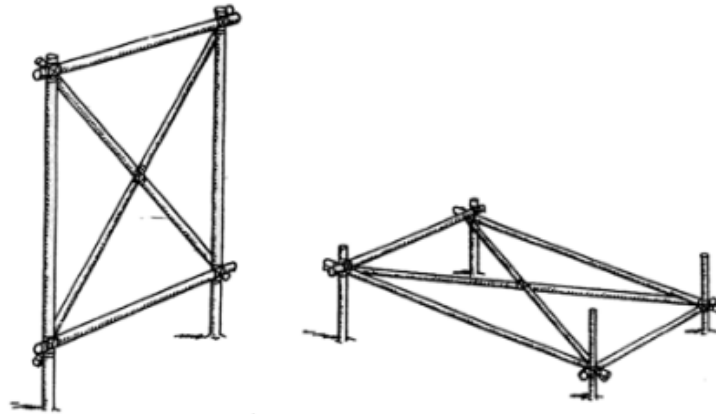
Figura 10. Recuadro horizontal y vertical para secar pieles.
